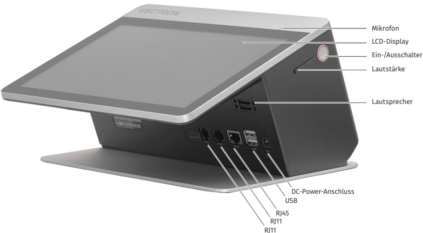
Abb. 1: Vorderansicht POS Life
