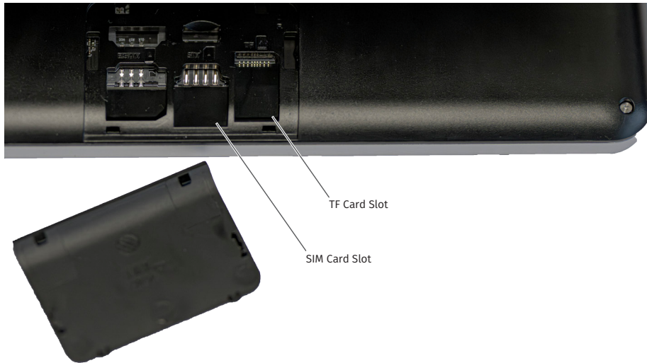
Abb. 3: Kartensteckplätze unter dem vorderen Displaygehäuse
