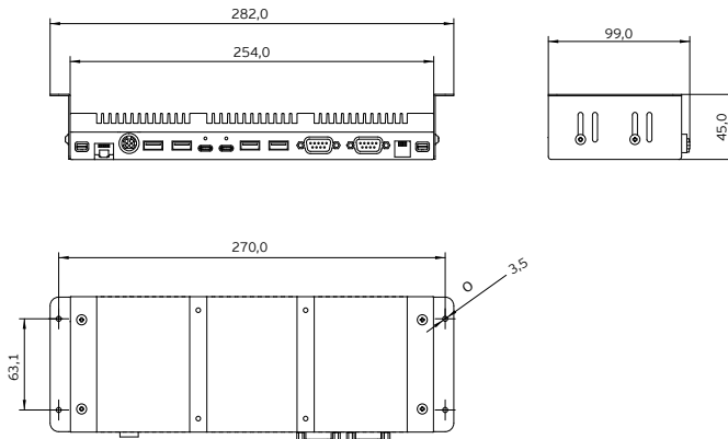
Abb. 11: Systembox inkl. Kühlkörper
