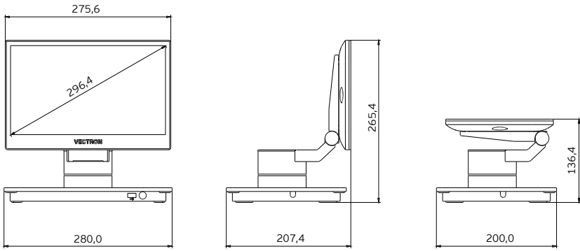
Abb. 9: Vectron POS 7 Mini Standfuß
