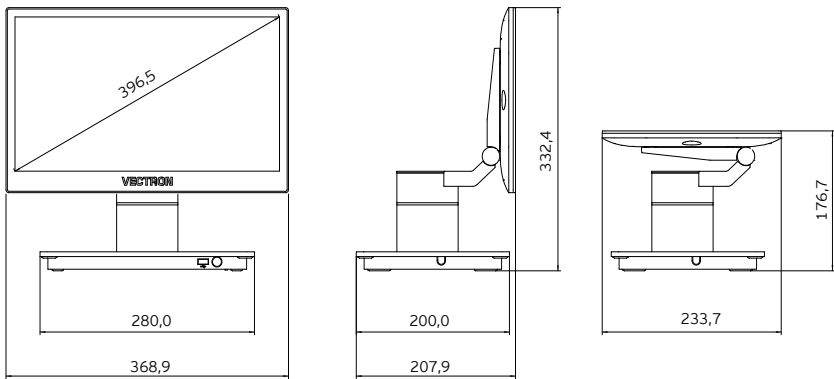
Abb. 7: Vectron POS 7 Standfuß
