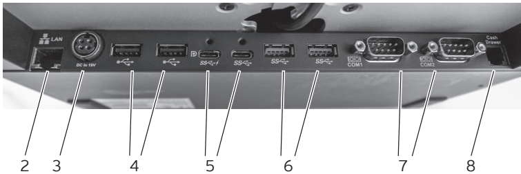
Abb. 5: Detailansicht der Schnittstellen und Anschlüsse POS 7 Standfuß
