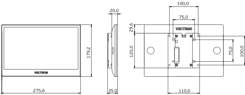
Abb. 10: Bedienerdisplay Vectron POS 7 Mini VESA an VESA Mount Adapter
