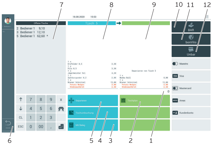
Abb. 20: Zahlungsoberfläche
