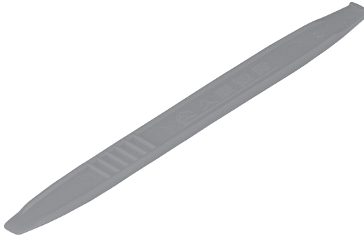
Abb. 29: Öffnungstool POS 7
